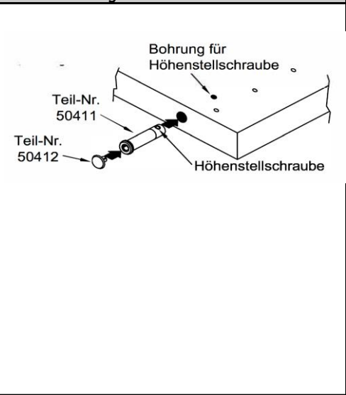
Abb. 2: Montage Höhenversteller
