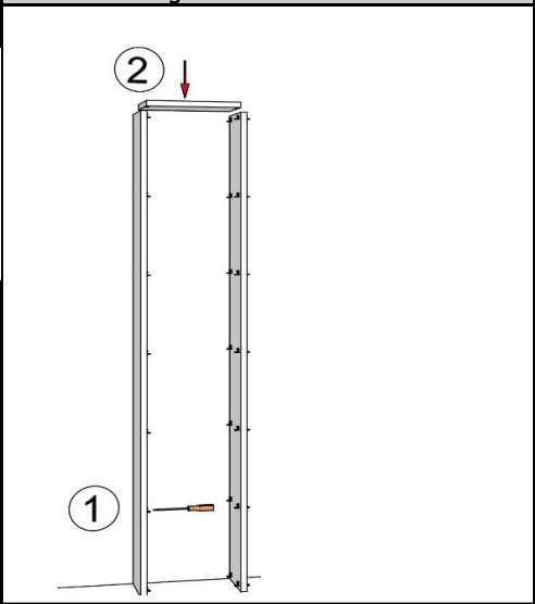
Abb. 3. Montage Stollen und -böden
